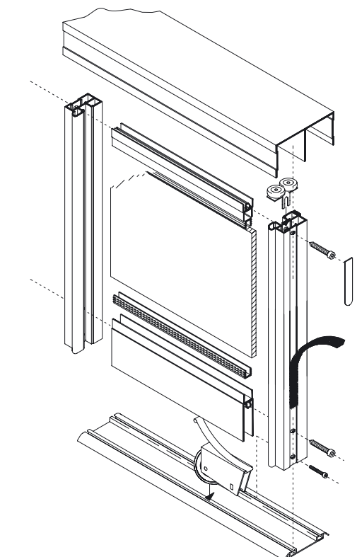
Sestav vrat 750/753
