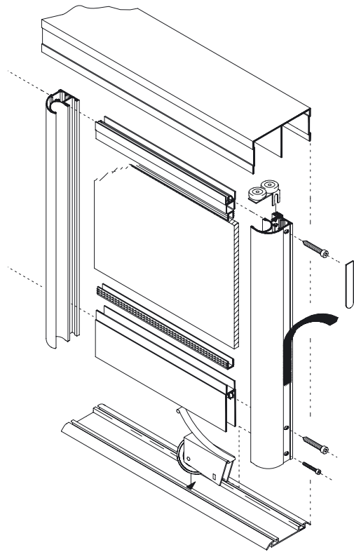
Sestav vrat 751
