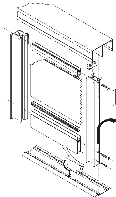
Sestav vrat 300
